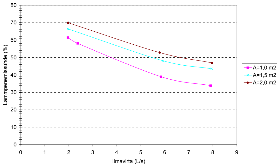
Kuva 3. Korvausilman lämpeneminen tuloilmaikkunassa tyypillisenä talvipäivänä. Korvausilma lämpenee ikkunan lämpöhäviön vaikutuksesta sekä auringonsäteilyn vaikutuksesta.
